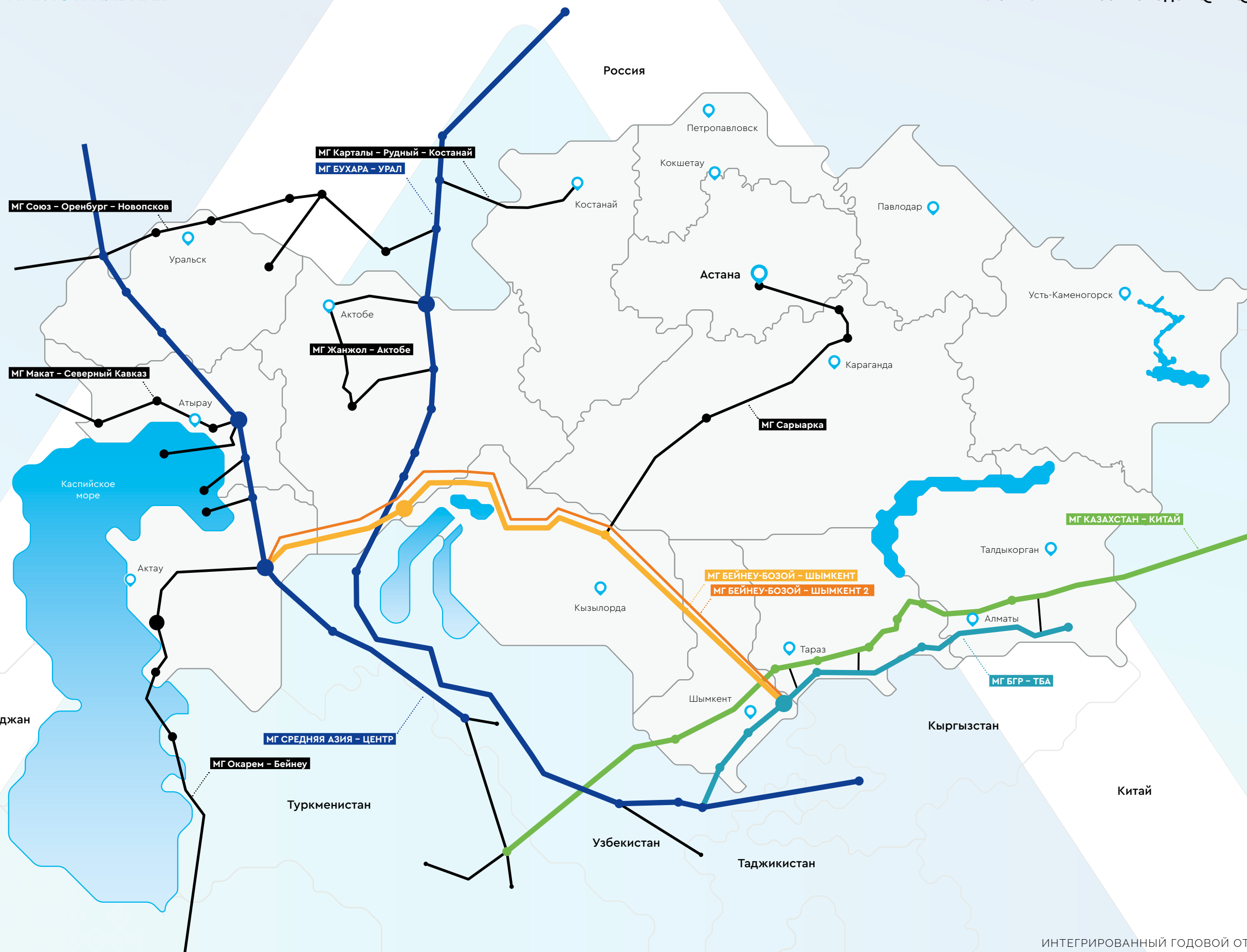
КАРТА МАГИСТРАЛЬНЫХ ГАЗОПРОВОДОВ QAZAQGAZ
