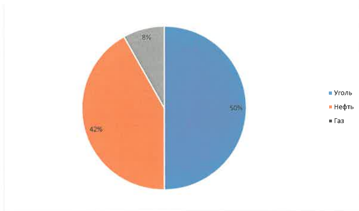
Рисунок 6. Выбросы ПГ по видам топлива за 2023 г. (MtCO 2 .)
