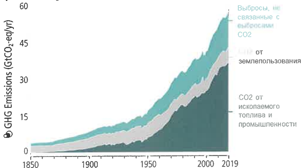
Рисунок 5. Выбросы ПГ, 1850-2019 гг.
