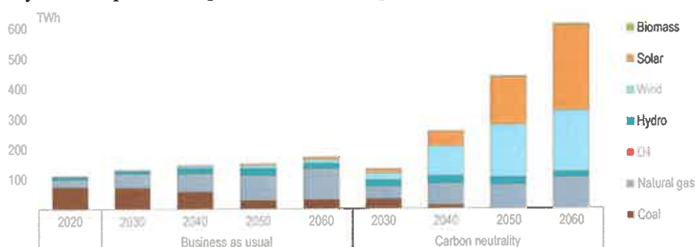
Рисунок 9. Прогнозы производства электроэнергии по сценариям, 2030-2060 гг.
